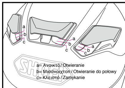
Πάνω εισαγωγή αέρα / Górný wlot powietrza
