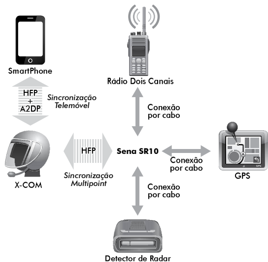
Conexão paralela do SR10 e telemóvel por
